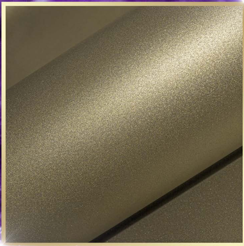
CR-11 Уваровит
