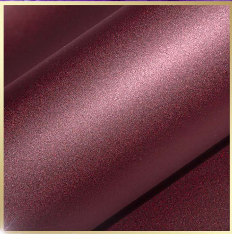
CR-09 Азурит
