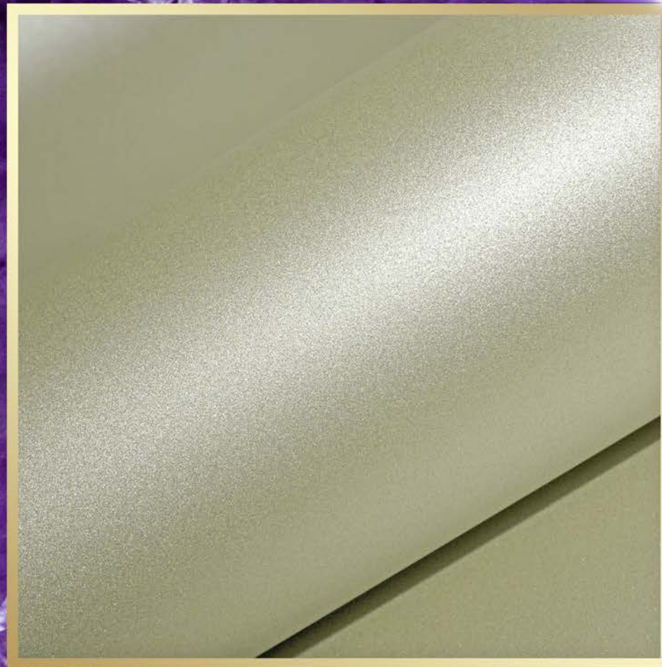
CR-06 Кальцит
