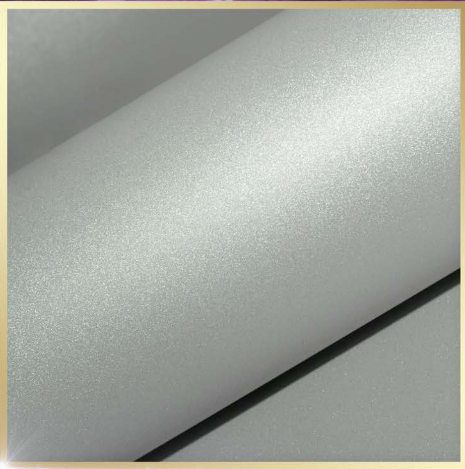
CR-01 Барит
