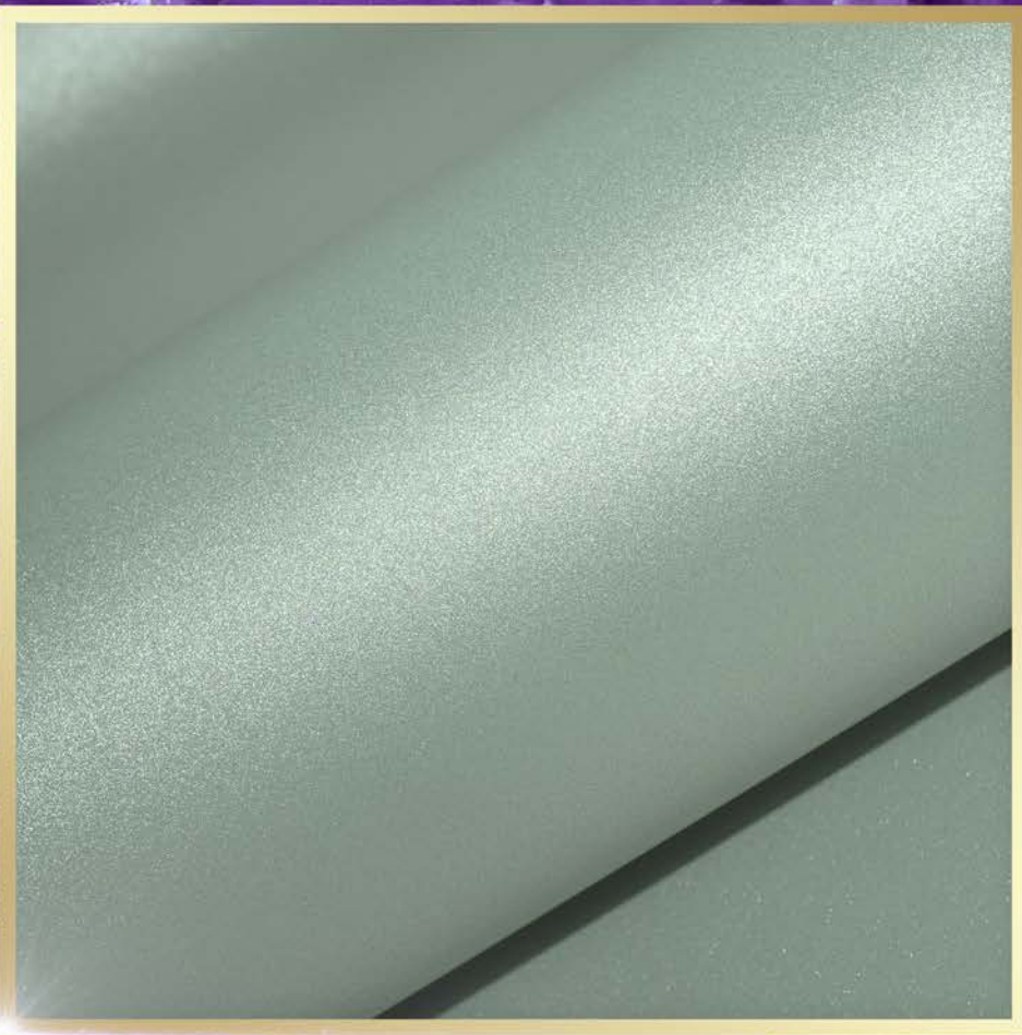
CR-07 Галенит
