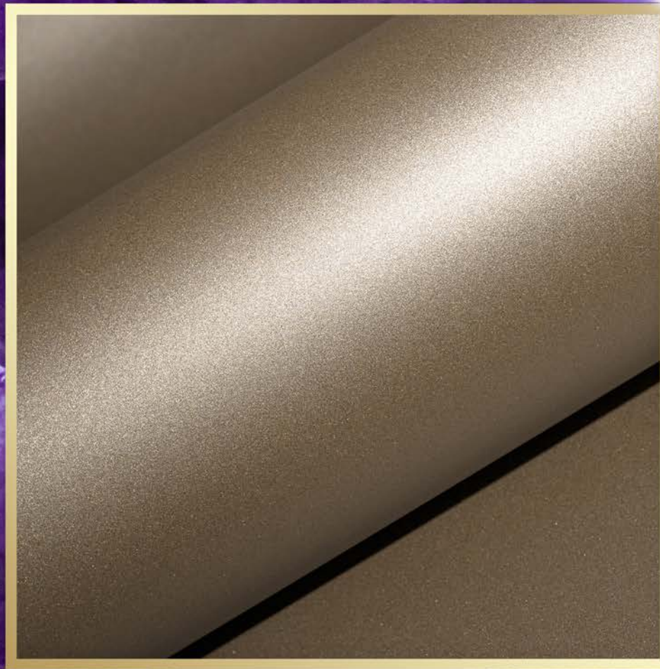
CR-08 Магнетит
