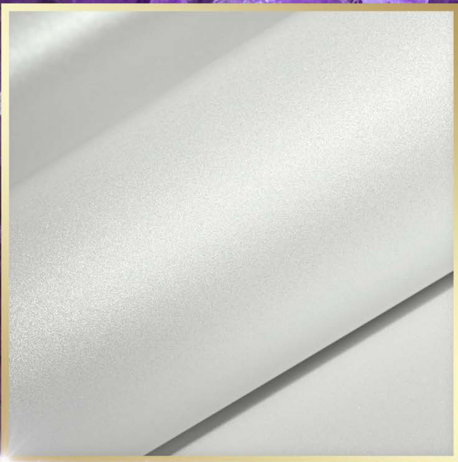
CR-03 Криолит
