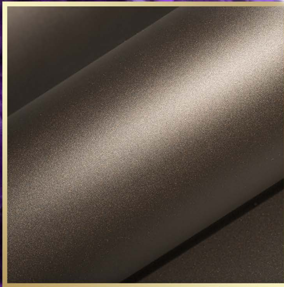
CR-10 Сидерит
